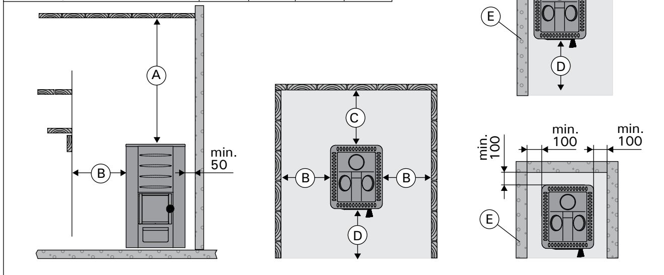
Obrázek 7. Bezpečné vzdálenosti pro topné těleso (všechny rozměry jsou uvedené v milimetrech)
