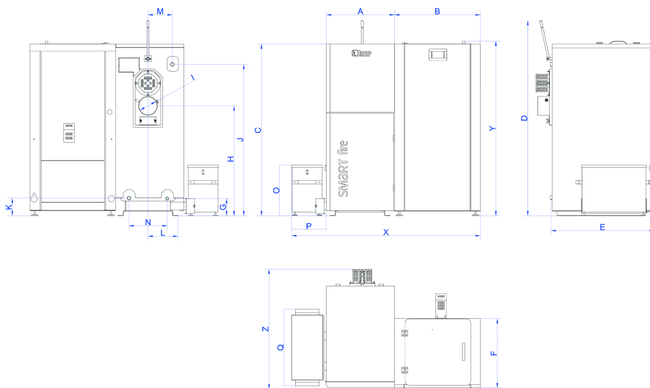
Rys nr 25. Wymiary kotłów Smart Fire SF31 oraz SF41 z zasobnikiem paliwa 240L i systemem automatycznego odpopielania
