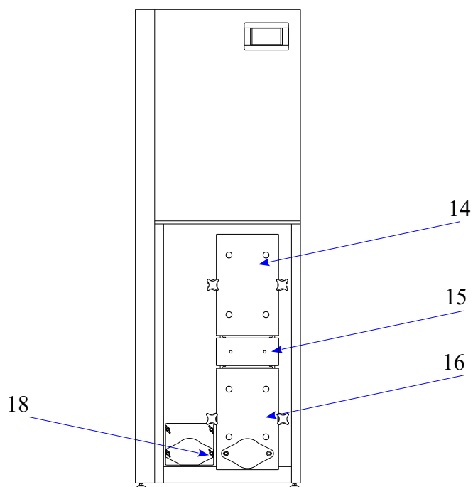
Rys nr 10. Opis schematyczny kotła Smart Fire SF11/130L 13-pokrywa otworu rewizyjnego; 14-drzwi komory spalania; 15-maskownica zapalarki ceramicznej oraz wyczystki palnika; 16-drzwi komory popielnika; 17-pokrywa otworu rewizyjnego czopucha spalinowego; 18-wyczystka dolnej części wymiennika ciepła;
