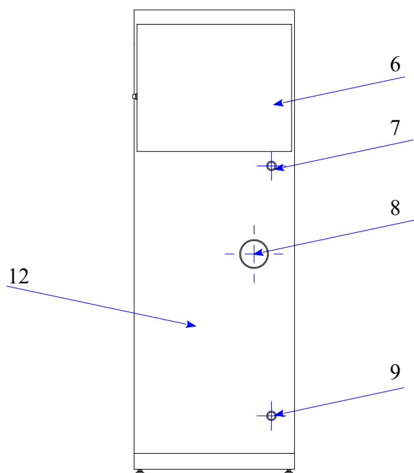
Rys nr 9. Opis schematyczny kotła Smart Fire SF11/130L 6-skrzynka elektryczna; 7-króciec zasilania; 8-czopuch spalinowy wraz z czujnikiem temperatury spalin oraz sondą Lambda (wyposażenie opcjonalne); 9-króciec wody powrotnej; 10-reset termostatu bezpieczeństwa STB (pod plastikową nakrętką); 11-pokrywa otworu rewizyjnego służą; 12-tylna maskownica;
