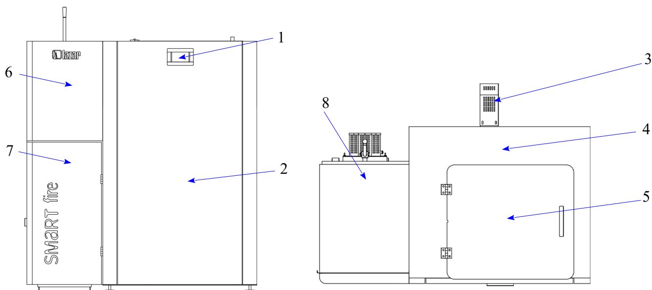
Rys nr 4. Opis schematyczny kotłów typu Smart Fire SF 11, SF15, SF15/3bar, SF22, SF22/3bar, SF31 oraz SF41:
