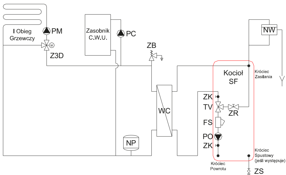
Rys nr 33. Układ zamknięty + CWU > 220L + 1 obieg na zaworze 3D
