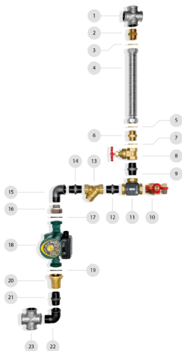
Rys nr 40. Zestaw hydrauliczny kotłów typu Smart Fire SF11 i SF15 1 ÷ 14 – jak na rys nr 29; 15-kolanko; 16-półśrubunek; 17-uszczelka gumowa; 18-pompa; 19-uszczelka gumowa; 20-półśrubunek z zaworem; 21-nypel; 22-kolanko; 23-czwórnik (przyłącze powrotu kotła);
