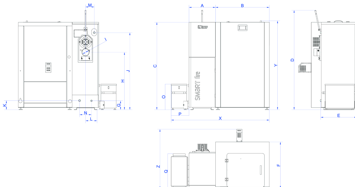
Rys nr 22. Wymiary kotłów Smart Fire SF11, SF15, SF15/3bar, SF22 oraz SF22/3bar z zasobnikiem paliwa 440L i systemem automatycznego odpopielania
