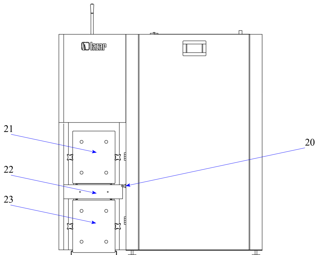
Rys nr 6. Opis schematyczny kotłów typu Smart Fire SF 11, SF15, SF15/3bar, SF22, SF22/3bar, SF31 oraz SF41 20-wyłącznik krańcowy maskownicy drzwi kotła; 21-drzwi komory palnika; 22-maskownica zapalarki ceramicznej oraz wyczystki palnika; 23-drzwi komory popielnika;
