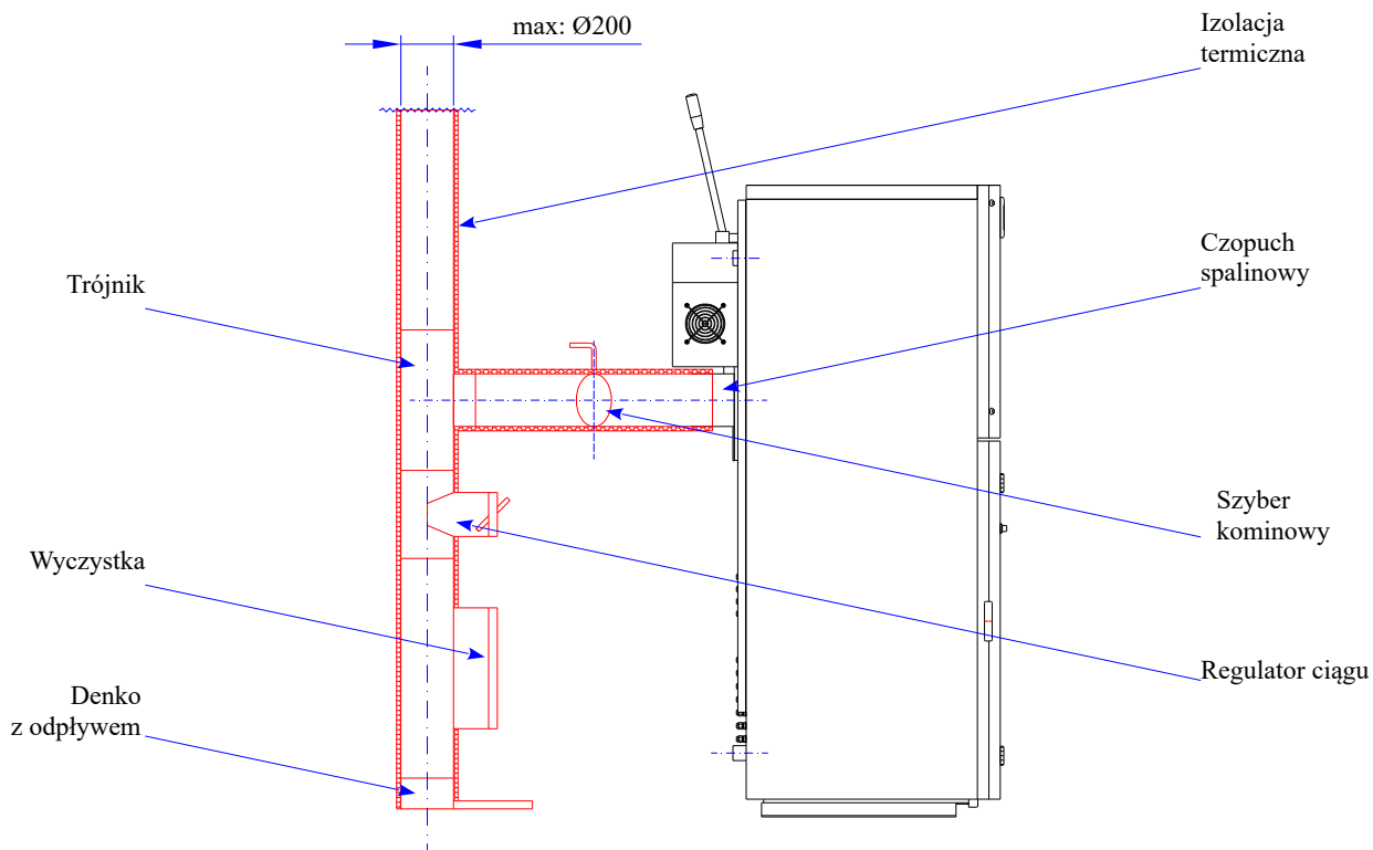
Rys nr 31. Przyłącze kominowe kotła Smart Fire
