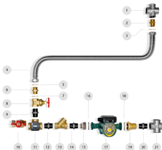
Rys nr 39. Zestaw hydrauliczny kotła typu Smart Fire SF11 z zasobnikiem 130L – SF11/130L: 1-czwórnik (przylącze zasilania kotła); 2-nypel mosiężny; 3-uszczelka twarda; 4-Przewód elastyczny EMICASA; 5-uszczelka twarda; 6-nypel mosiężny; 7-uszczelka twarda; 8-zawór zasurowy (kryzujący); 9-nypel; 10-zawór kulowy (przylącze powrotu instalacji); 11-zawór termostatyczny TV 55°C; 12-nypel; 13-filtr; 14-nypel; 15-półśrubunek; 16-uszczelka gumowa; 17-pompa; 18-uszczelka gumowa; 19-półśrubunek z zaworem; 20-nypel; 21-czwórnik (przylącze powrotu kotła);
