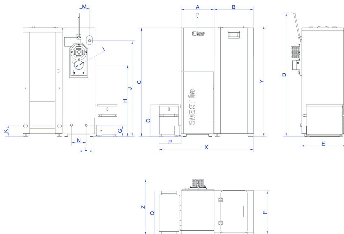
Rys nr 20. Wymiary kotłów Smart Fire SF11, SF15, SF15/3bar, SF22 oraz SF22/3bar z zasobnikiem paliwa 150L i systemem automatycznego odpowielania
