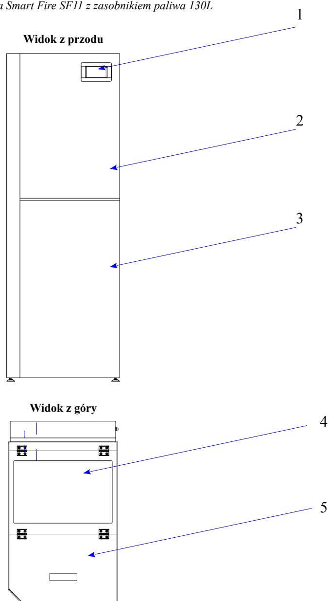
Rys nr 8. Opis schematyczny kotła Smart Fire SF11/130L
