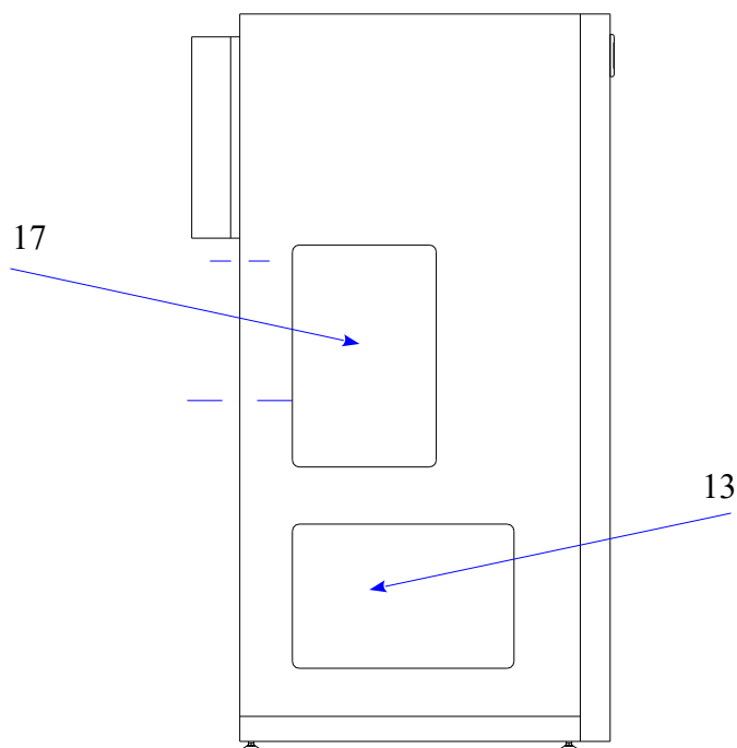
Rys nr 10. Opis schematyczny kotła Smart Fire SF11/130L 13-pokrywa otworu rewizyjnego; 14-drzwi komory spalania; 15-maskownica zapalarki ceramicznej oraz wyczystki palnika; 16-drzwi komory popielnika; 17-pokrywa otworu rewizyjnego czopucha spalinowego; 18-wyczystka dolnej części wymiennika ciepła;
