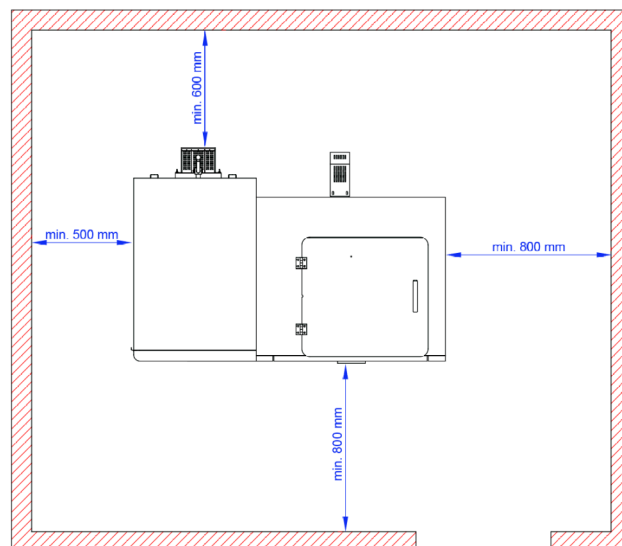
Rys nr 30. Przykład umiejscowienia kotła typu Smart Fire SF41 z zasobnikiem 440L w kotłowni
