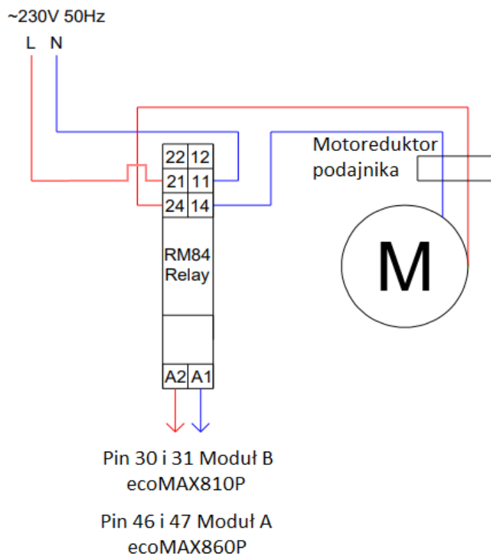
Rys nr 19. Schemat podłączenia systemu automatycznego odpopielania do regulatora kotła.
