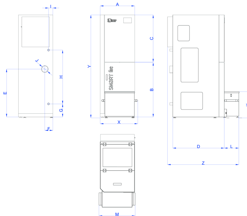
Rys nr 23. Wymiary kotła Smart Fire SF11 z zasobnikiem paliwa 130L i systemem automatycznego odpowielania
