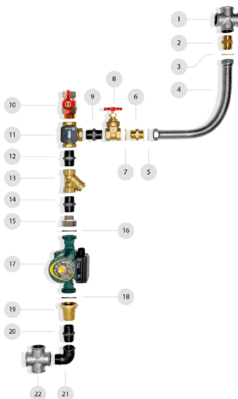
Rys nr 41. Zestaw hydrauliczny kotłów typu Smart Fire SF15/3bar, SF22, SF22/3bar, SF31 oraz SF41: 1-czwórnik (przyłącze zasilania kotła); 2-nypel mosiężny; 3-uszczelka twarda; 4-Przewód elastyczny EMICASA; 5-uszczelka twarda; 6-nypel mosiężny; 7-uszczelka twarda; 8-zawór zasuwny (kryżujący); 9-nypel; 10-zawór kulowy (przyłącze powrotu instalacji); 11-zawór termostatyczny TV 55°C; 12-nypel; 13-filtr; 14-nypel; 15-półśrubunek; 16-uszczelka gumowa; 17-pompa; 18-uszczelka gumowa; 19-półśrubunek z zaworem; 20-nypel; 21-kolanko; 22-czwórnik (przyłącze powrotu kotła);
