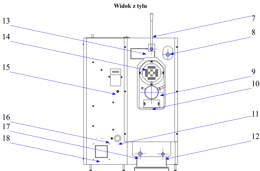
Rys nr 17. Opis schematyczny kotłów typu Smart Fire SF 11, SF15, SF15/3bar, SF22, SF22/3bar, SF31 oraz SF41: 7-dźwignia mechanizmu czyszczenia wymiennika; 8-króciec wody grzewczej; 9-czopuch spalinowy wraz z czujnikiem temperatury spalin oraz sondą Lambda (wyposażenie opcjonalne); 10-wyczystka kolektora spalin; 11-przepust dla okablowania; 12-króciec spustowy; 13-punkt montażu układu napędowego automatycznego systemu czyszczenia wymiennika (wyposażenie opcjonalne); 14-obudowa wentylatora wyciągowego; 15-reset termostatu bezpieczeństwa (pod plastikową nakrętką); 16-dławnica kabla zasilającego; 17-króciec wody powrotnej; 18-punkt montażu systemu zewnętrznej dystrybucji powietrza;
