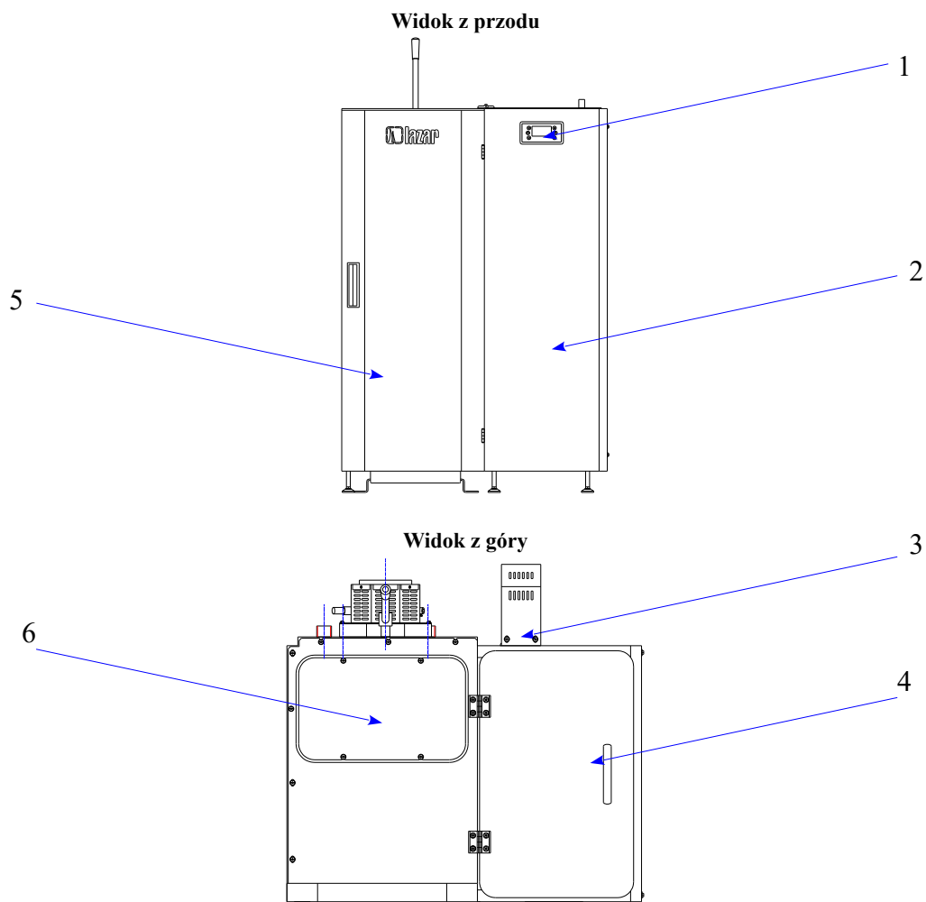
Rys nr 16. Opis schematyczny kotłów typu Smart Fire SF 11 Compact oraz SF15 Compact: 1-panel wyświetlacza dotykowego; 2-zasobnik paliwa; 3-obudowa układu napędowego ślimaka zasobnika paliwa; 4-klapa zasobnika paliwa; 5-maskownica drzwi kotła; 6-pokrywa rewizyjna pokrywy górnej części wymiennika ciepła;
