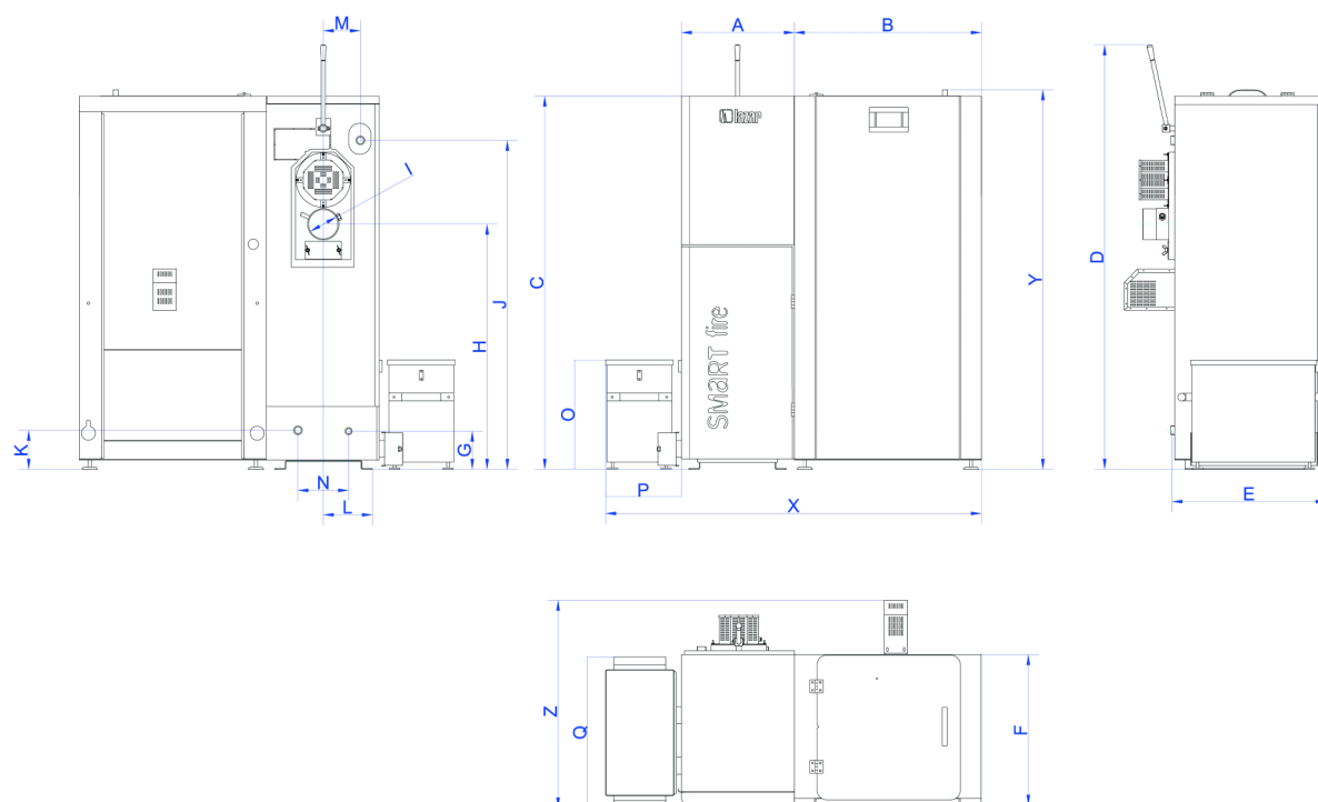
Rys nr 21. Wymiary kotłów Smart Fire SF11, SF15, SF15/3bar, SF22 oraz SF22/3bar z zasobnikiem paliwa 240L i systemem automatycznego odpowielania
