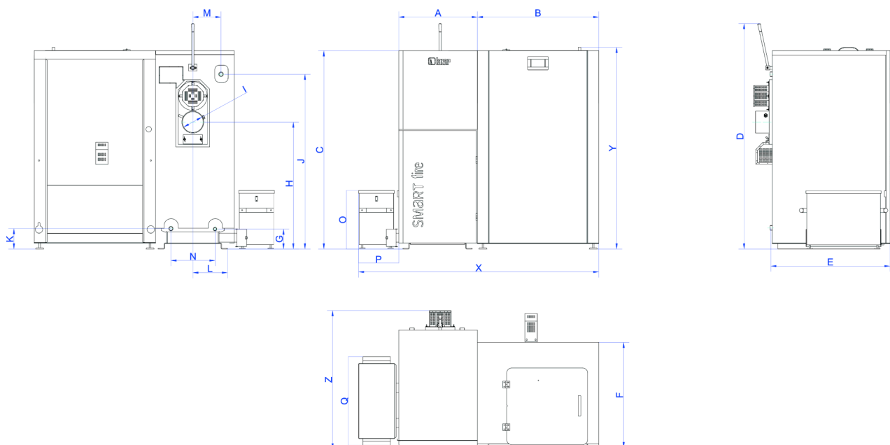
Rys nr 26. Wymiary kotłów Smart Fire SF31 oraz SF41 z zasobnikiem paliwa 440L i systemem automatycznego odpowielania
