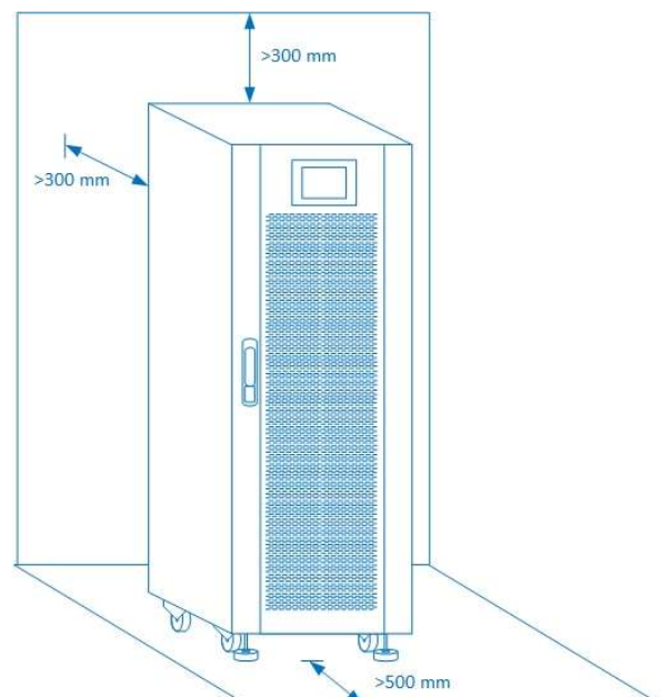
Rys. 3-1. Wymiary zalecanej przestrzeni serwisowej
