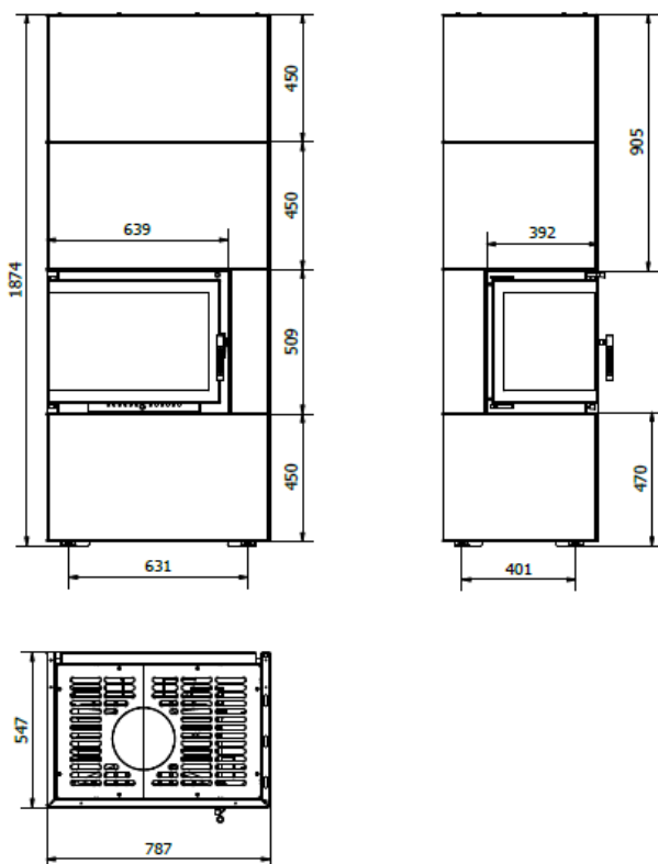
Rys. 2. Zwymiarowany rysunek zabudowy SIMPLE BOX w wersji BSL
