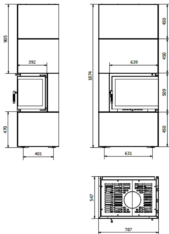
Rys. 1. Zwymiarowany rysunek zabudowy SIMPLE BOX w wersji BSP
