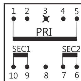
TEZ 20; 25; 30
