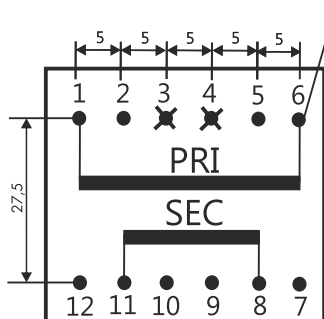
TEZ 10
