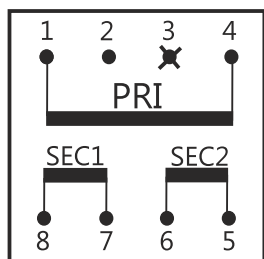
TEZ 16
