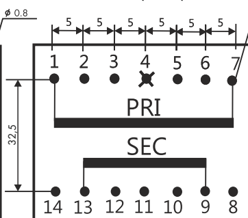
TEZ 20; 25; 30
