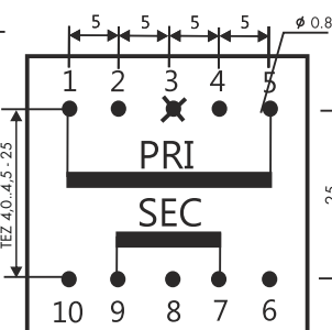
TEZ 1,5 - 4,5
