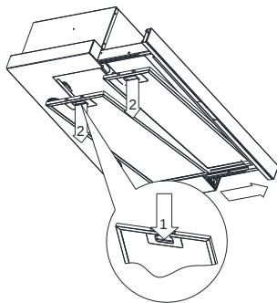
Rys. 4 Demontaż filtrów aluminiowych przeciw tłuszczowych
