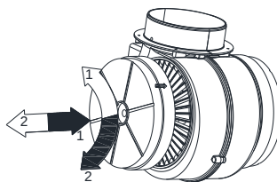
Rys. 7 Wymiana filtra węglowego.
