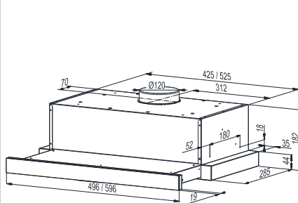
Rys. 2 Rysunek gabarytowy.
