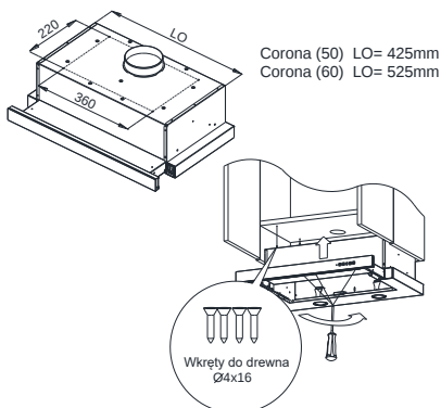
Rys. 5d Montaż korpusu okapu wersja mocowanie górne.
