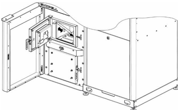
KROK 3. Oczyszczyć powierzchnię rusztu i ściany boczne paleniska oraz wnętrze komory paleniskowej.
