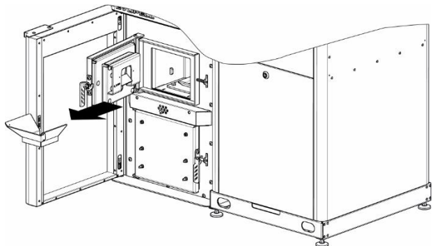
KROK 2. Wyjąć zsyg paleniska.
