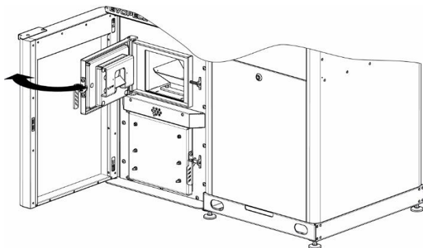
KROK 1. Otworzyć drzwi osłonowe oraz drzwi paleniskowe
