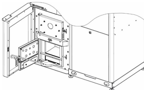
KROK 3. Oczyszczyć dno komory nawrotnej i tunel wentylatora spalin.
