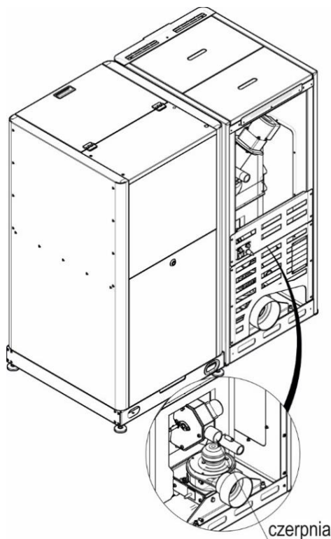
Rysunek 12. Czerpnia powietrza - otwór dolotowy powietrza.
