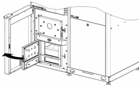
KROK 1. Otworzyć drzwi osłonowe oraz drzwi popielnikowe
