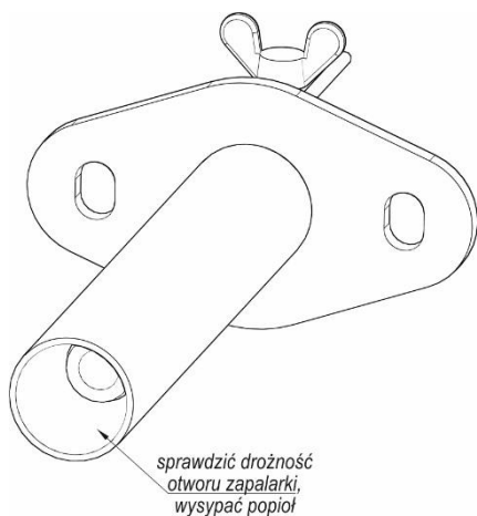
Rysunek 17. Sposób czyszczenia otworu zapalarki
