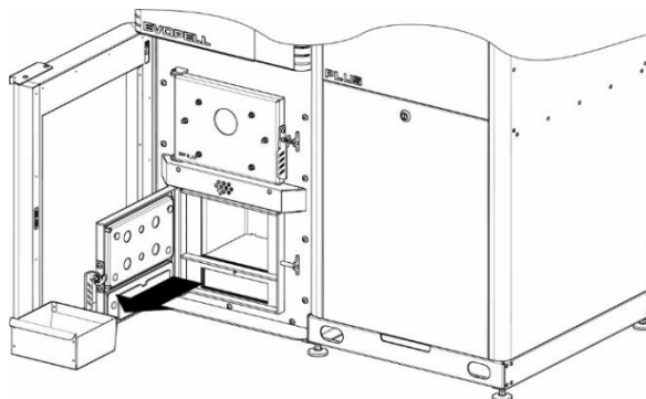
KROK 2. Wysunąć pojemnik na popiół i usunąć popiół.
