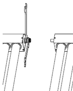
Zasada skręcania złązek
