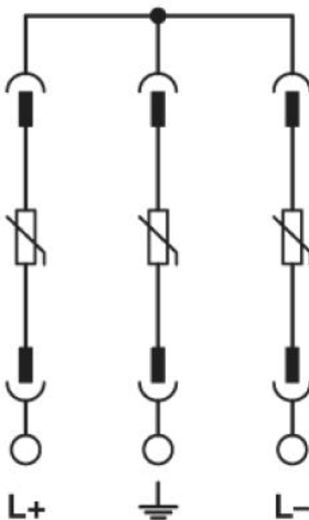
Schemat
