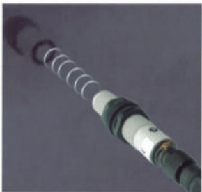
超声波传感器 Ultrasonic sensor RU18系列 RU18 Series
