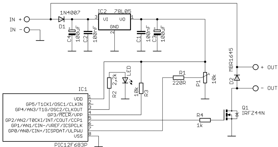
Rys. 1. Schemat ideowy
