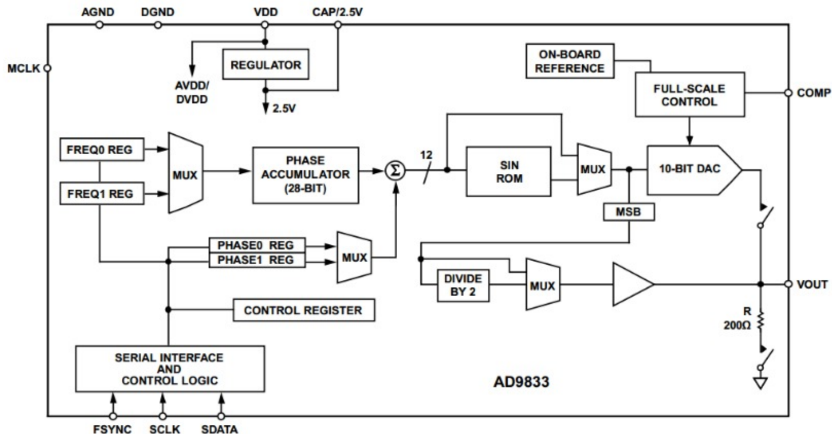
schemat blokowy wewnętrznej budowy AD9833:
