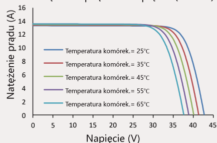
Natężenie prądu – Napięcie (475 W)
