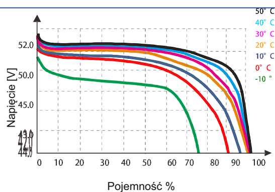
Krywa rozładowania w różnych temperaturach (0,5C)
