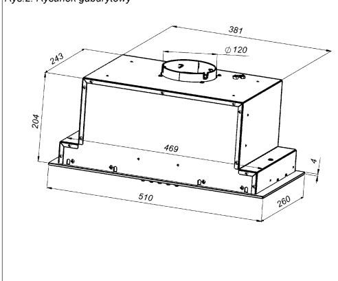
Rys. 2: Rysunek gabarytowy
