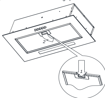
Rys.: 6b Montaż okapu - wersja mocowania boczna
