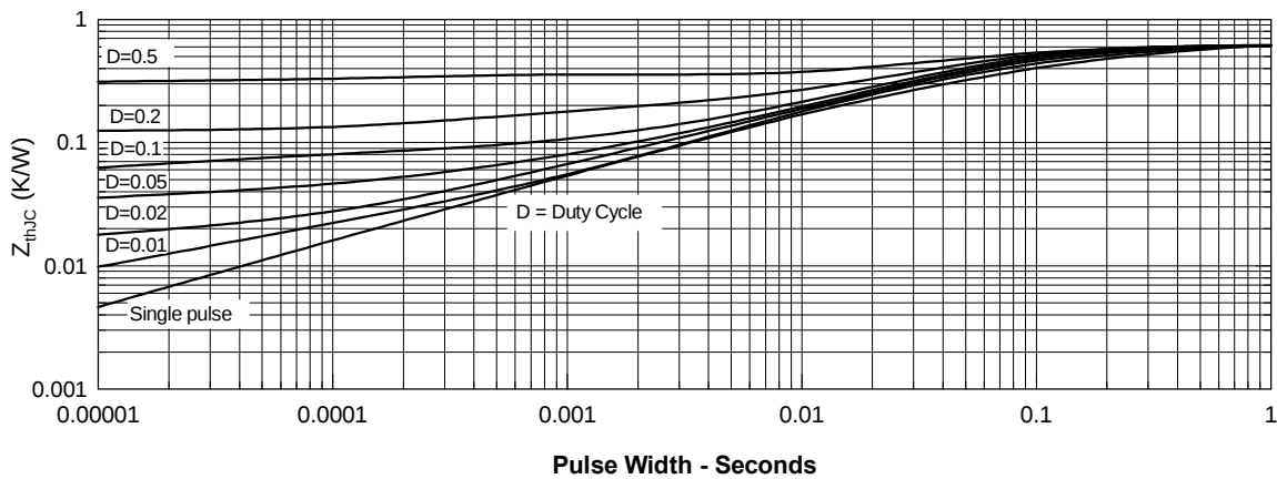
Fig. 10. Thermal Impedance
