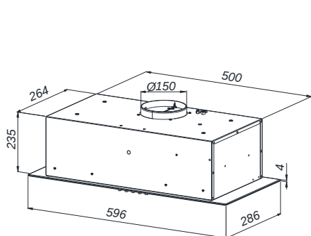
Rys. 2 Rysunek gabarytowy.
