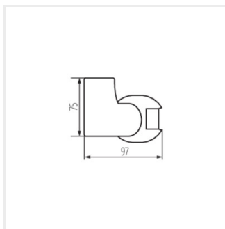
ALER JQ-30
