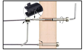
Stap6. Draai ten slotte de schroef met de gebogen sleutel om vast te draaien de spanner en het geheel kabel apparaat .
