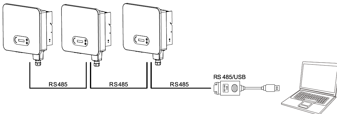
Rysunek 4-20: Podłączanie przewodów komunikacyjnych w przypadku wielu falowników SOFAR 3.3~12KTLX-G3
