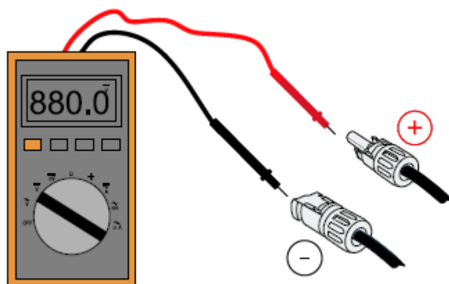
Rysunek 4-14 Podłączanie przewodu prądu stałego (4)
