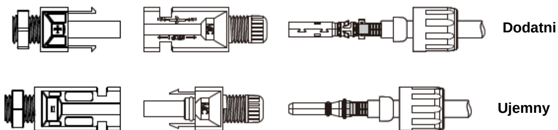
Rysunek 4-14 Podłączanie przewodu prądu stałego (4)
