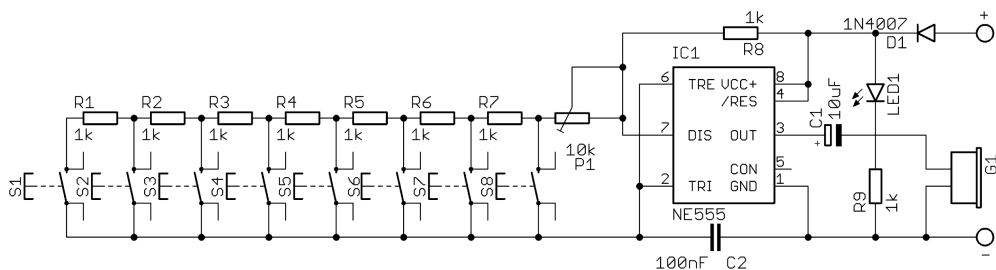
Rys. 1. Schemat ideowy
