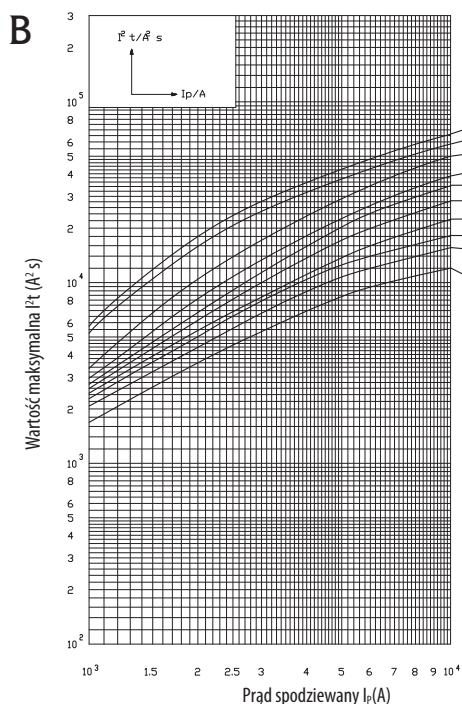
Charakterystyki całek wyłączenia I^2t wyłączników - charakterystyki B, C, D, K
