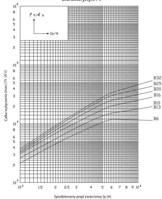
Charakterystyki I^2t
