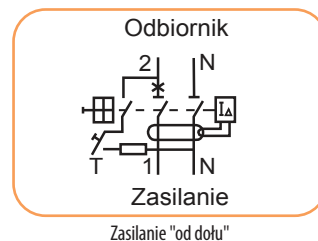
Układ połączeń - wewnętrzny
