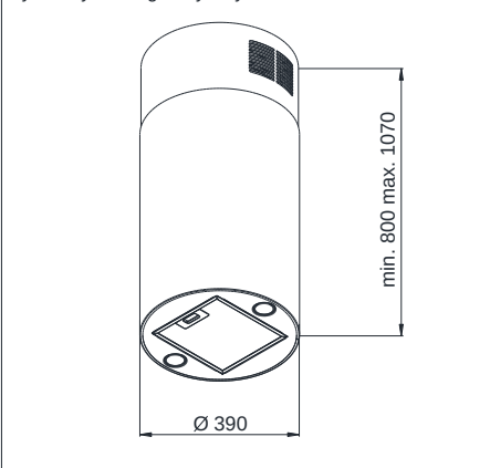
Rys. 2 Rysunek gabarytowy.
