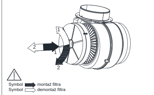
Rys. 9 Wymiana filtra węglowego.
