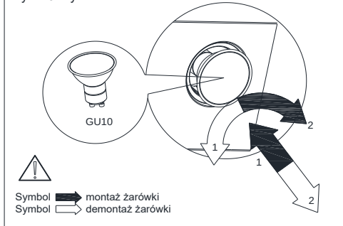
Rys. 10 Wymiana oświetlenia.
