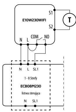
c) Schemat podłączenia do listwy sterującej
