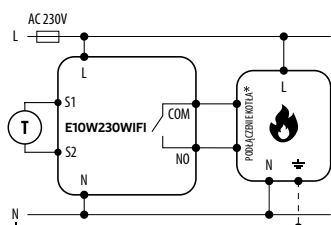
a) Schemat podłączenia do kotła gazowego
