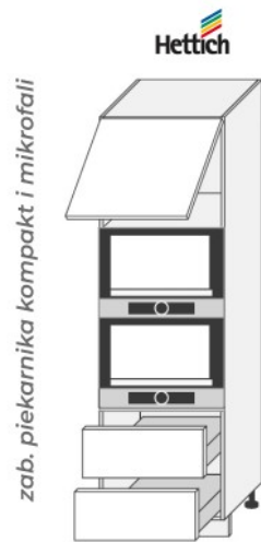
D14 RU 2A KOMPACT (600/2070/565)
