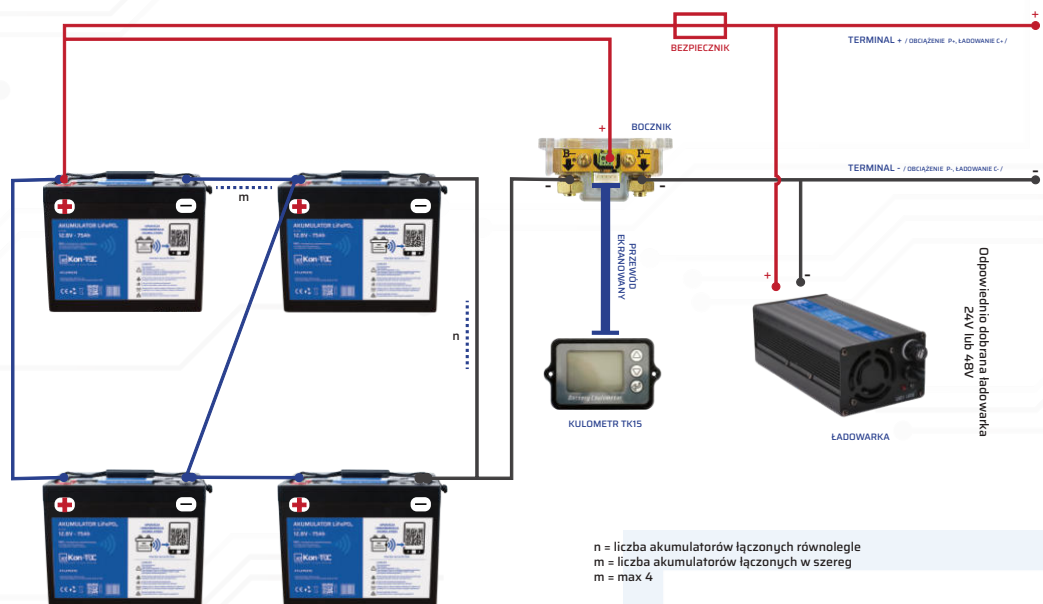
Rys.5. Schemat szeregowo-równoległego połączenia akumulatorów
