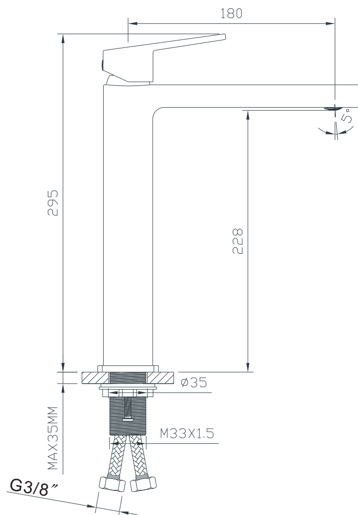
RYSUNEK TECHNICZNY
