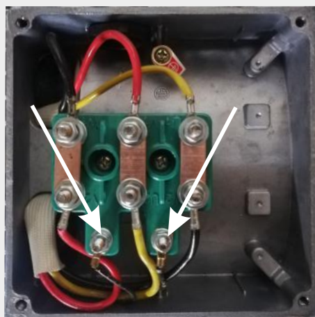
Rys. 2. Skrzynka podłączeniowa silnika trójfazowego / Fig. 2. Three-phase motor connection box
