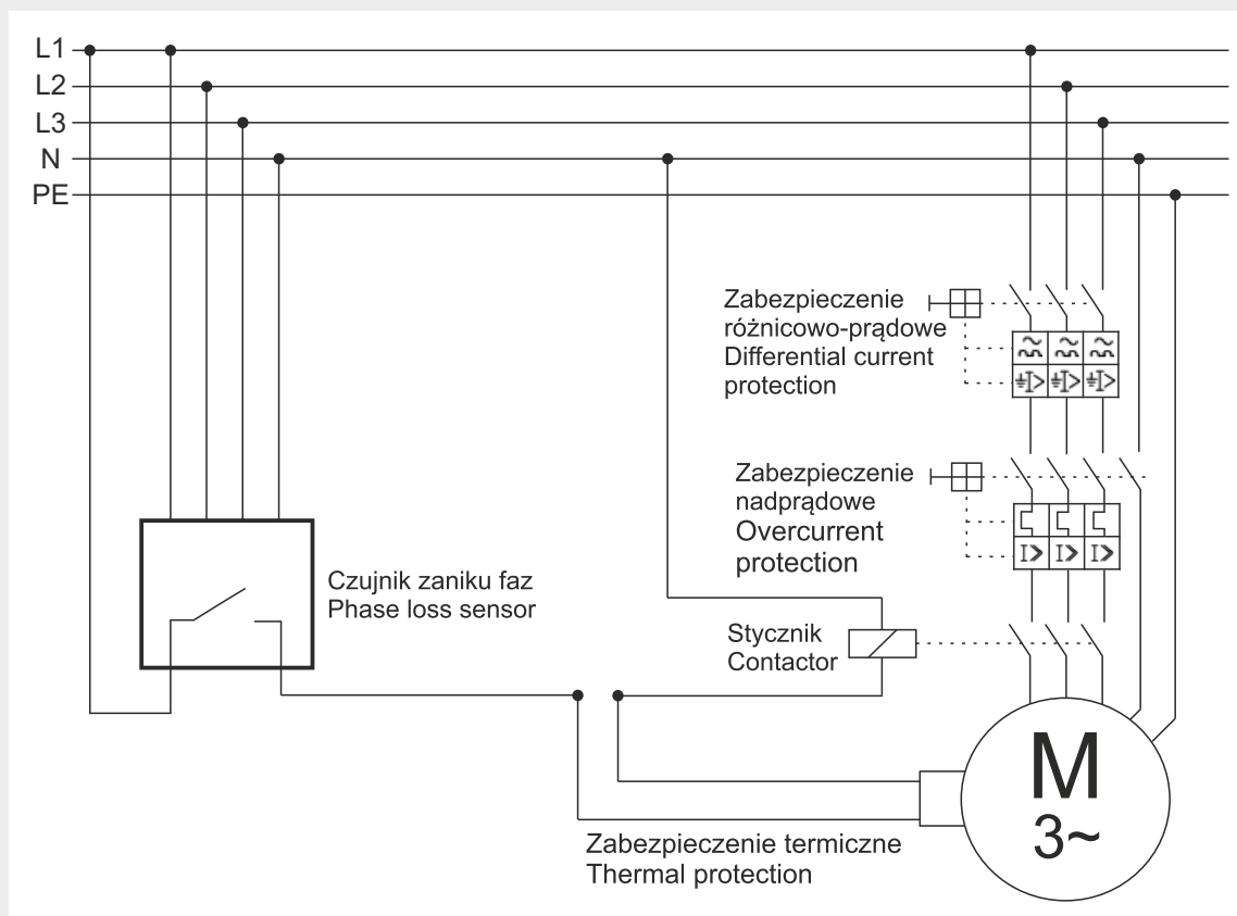
Rys. 3. Przykładowy schemat podłączenia silnika trójfazowego / Fig. 3. Three-phase motor connection diagram
