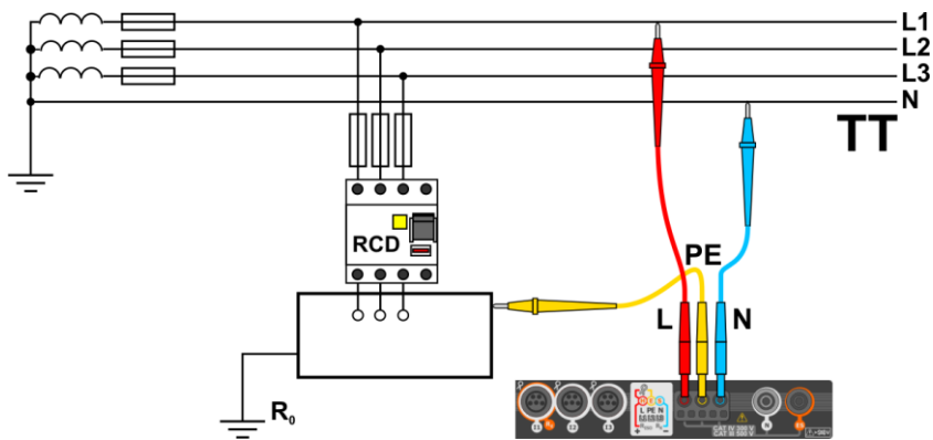
Rys. 3.4 Pomiar w układzie TT
