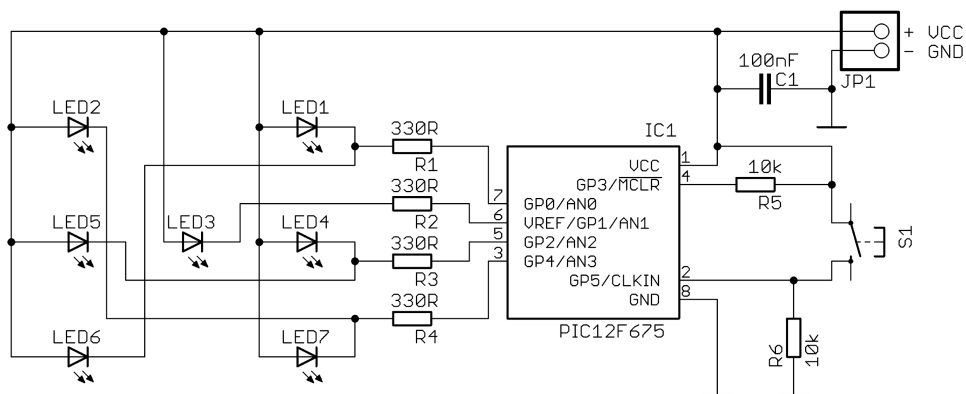
Rys. 2 Schemat ideowy
