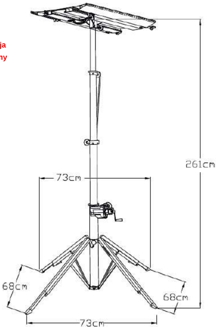
Składana rama aluminiowa do płyt GK i paneli
