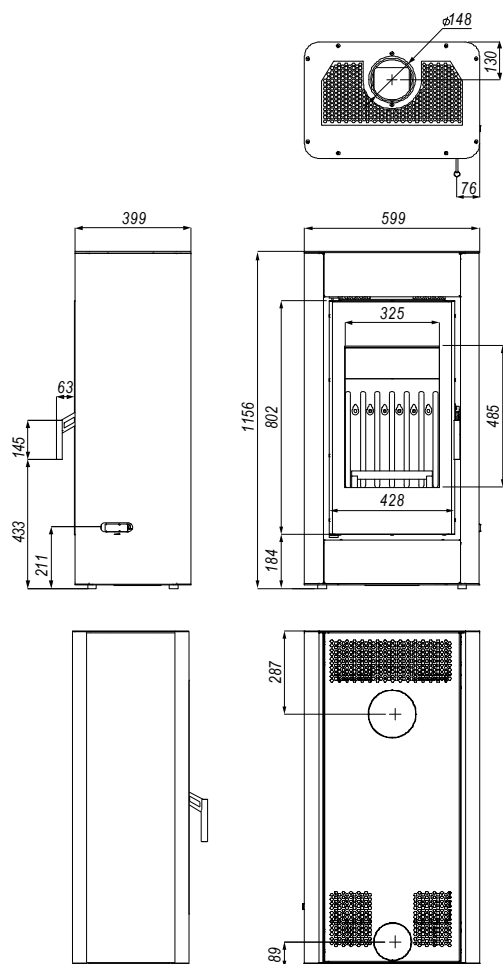
Rysunek 3. Wymiary (w mm) pieca wolnostojącego serii IGNIS w wersji SOLUM BOX.
