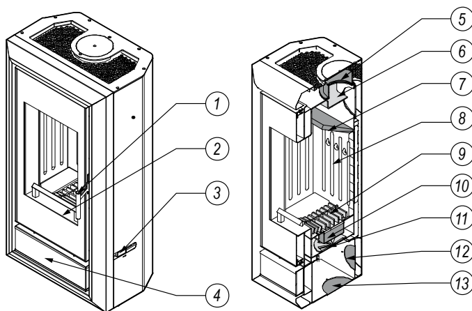
Rysunek 1. Budowa pieca wolnostojącego serii IGNIS.
