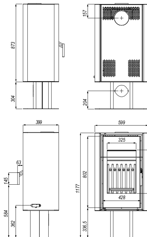
Rysunek 5. Wymiary (w mm) pieca wolnostojącego serii IGNIS w wersji SOLUM TOP.
