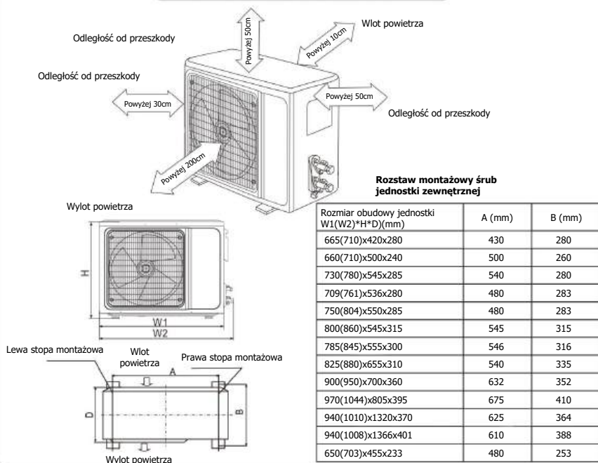
Rysunek wymiarowy instalacji jednostki zewnętrznej
