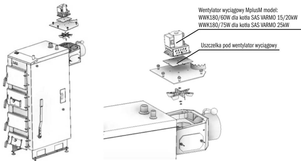
Rysunek 3. Wentylator wyciągowy (wyposażenie dodatkowe) – montaż bezpośrednio w czopuchu kotła SAS VARMO 15/20/25 kW
