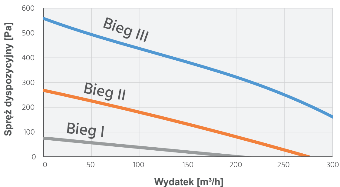
izzI V.302 ERV (300 m³/h; 150 Pa)
