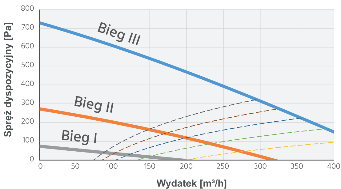
izzI V.402 ERV (400 m³/h; 150 Pa)
