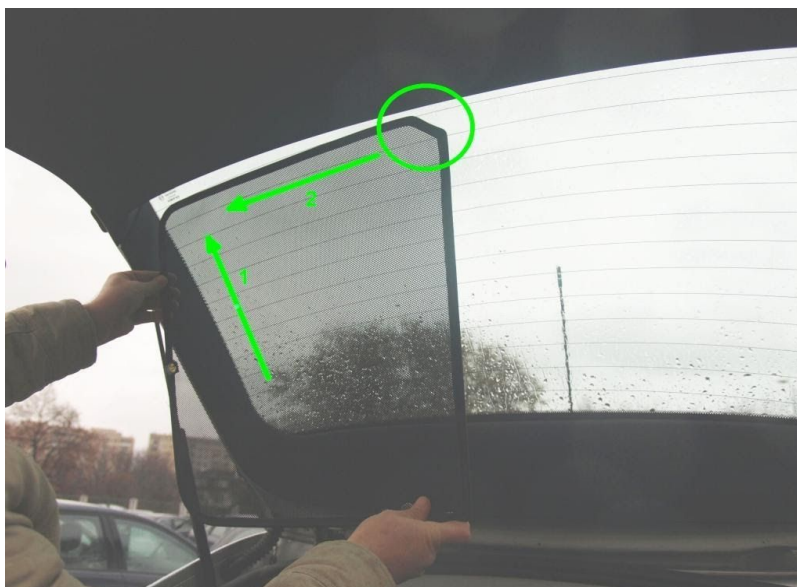
Zdjęcie nr 5 - Montaż zasłonek klapy bagażnika
