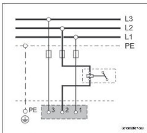
Fig. 41 Schéma de câblage
