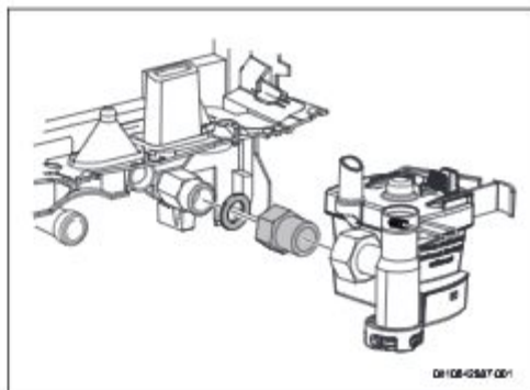
Rys. 28 Dodatkowa tuleja
