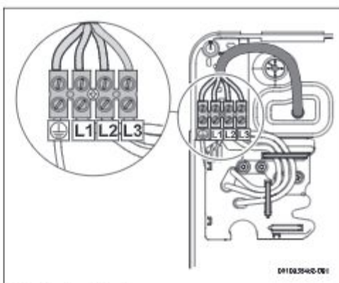
Bild 43 Anschluss oben
