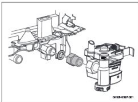
Bild 29 Zusätzliche Buchse
