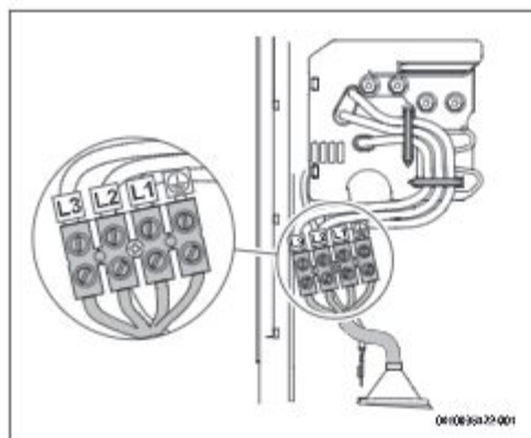
Bild 44 Anschluss unten
