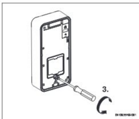
Rys. 10 Wykreślenie śruby
