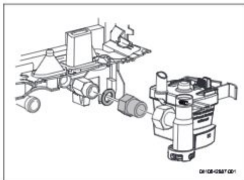
Fig. 28 Bague supplémentaire
