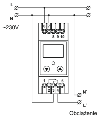
Schemat połączeń
