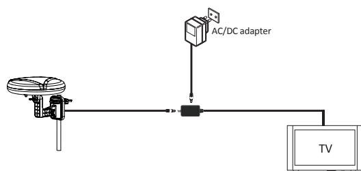
Schemat podłączenia anteny do TV z wbudowanym tunerem DVB-T/T2
