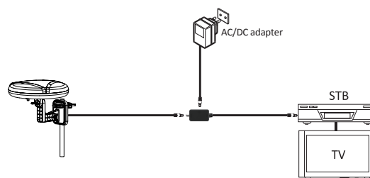
Schemat podłączenia anteny do tunera DVB-T/T2 zewnętrznego
