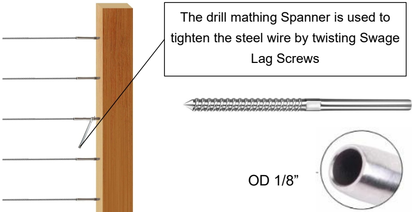
Accesorio para poste de madera
