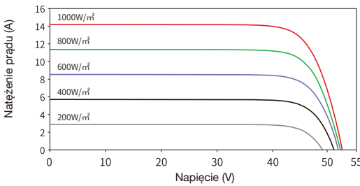
Wykres prądu w funkcji napięcia (72HL4-(V) 595W)
