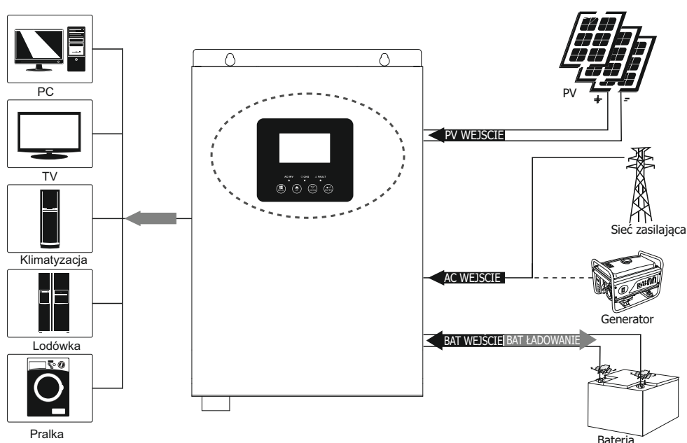
Rys 1. Hybrydowy system zasilania
