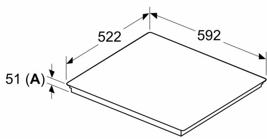
Wymiary w mm
