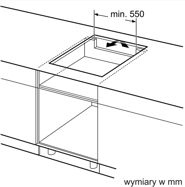
A: Głębokość wpuszczenia
