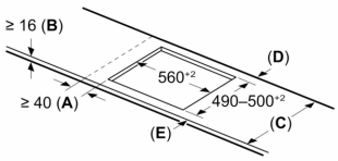
Wymiary w mm
