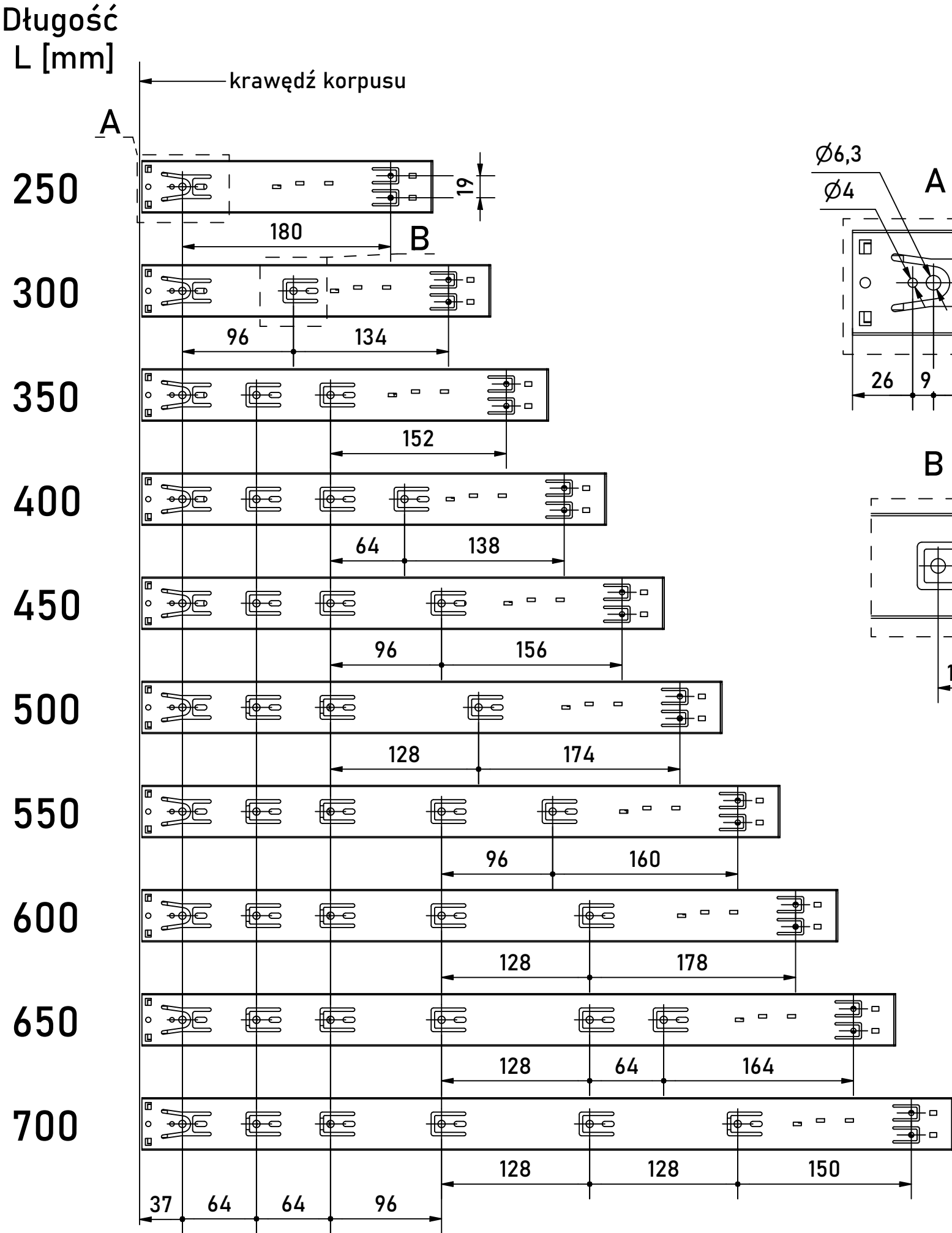
Widok na boku korpusu
