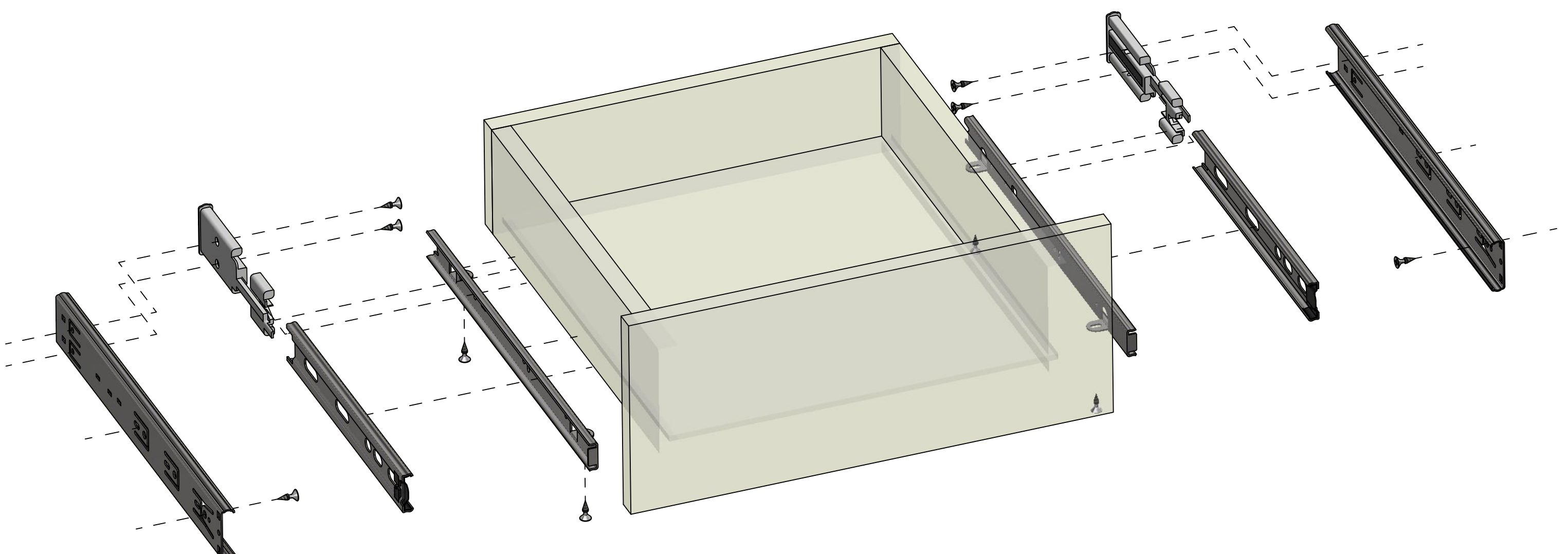
Montaż prowadnic do szuflady i korpusu
