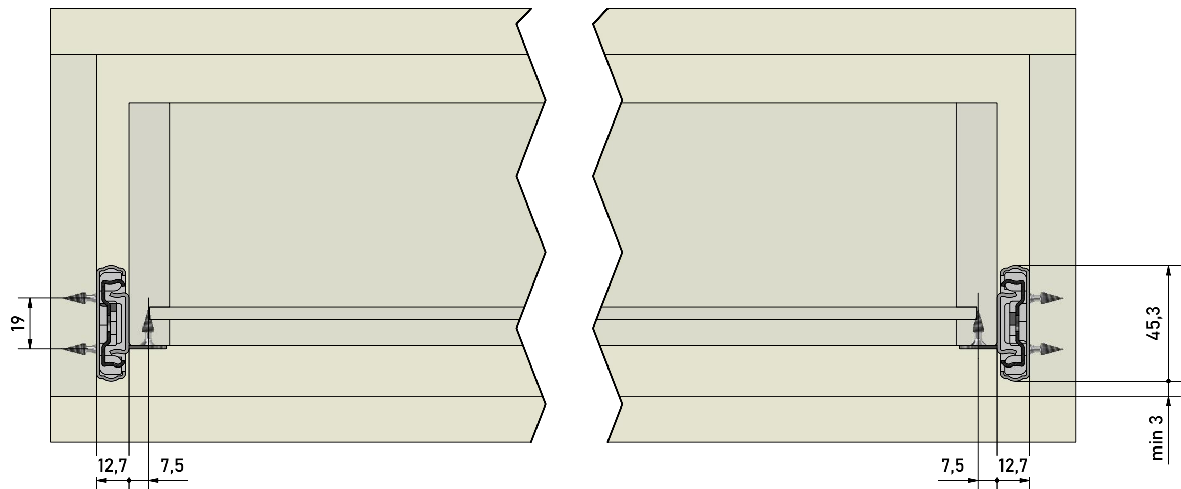
Widok szuflady od spodu
