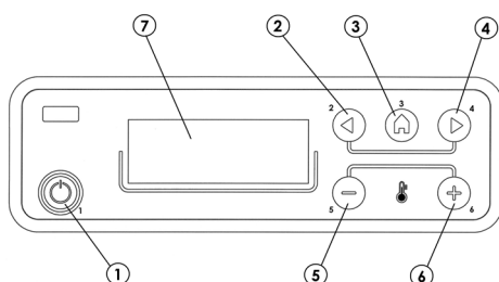
Fig. 2 - Panel sterowania
