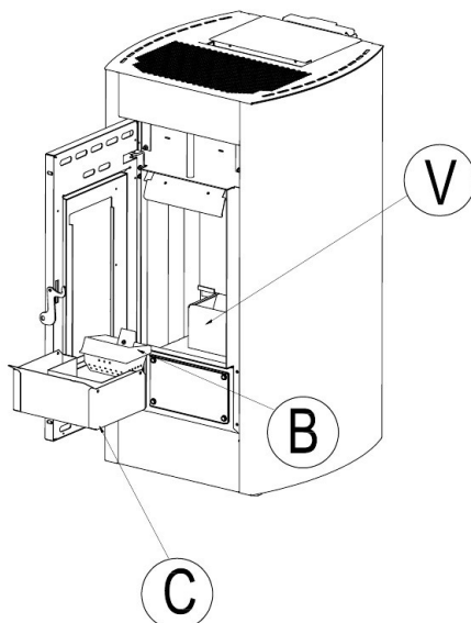
Fig. 22 - Czyszczenie
