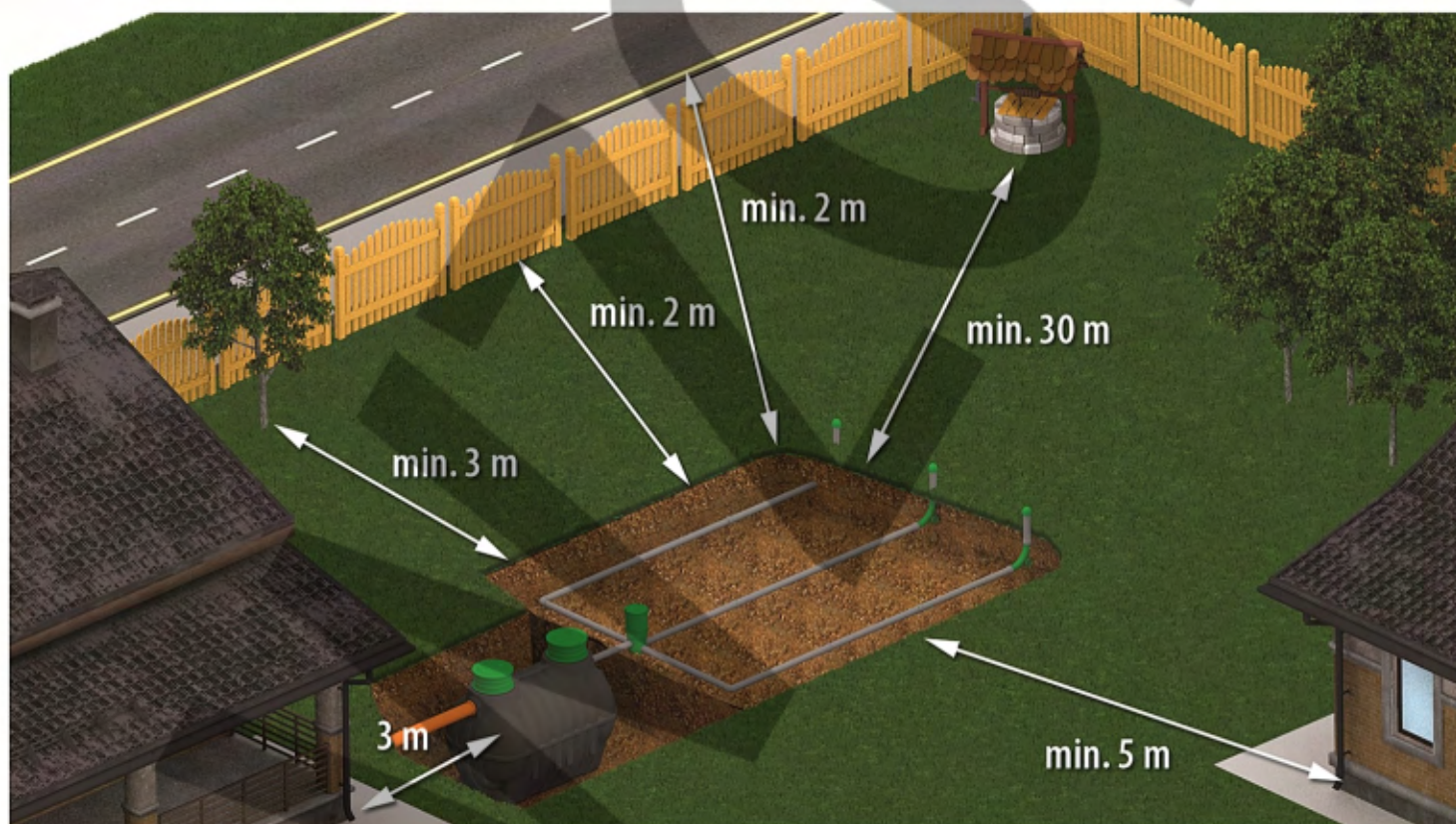
Rys. 8. Lokalizacja oczyszczalni wymagania
