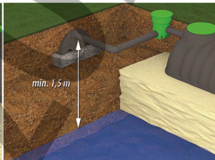
Rys. 7. Odległość ochronna / Tunel rozsączający
