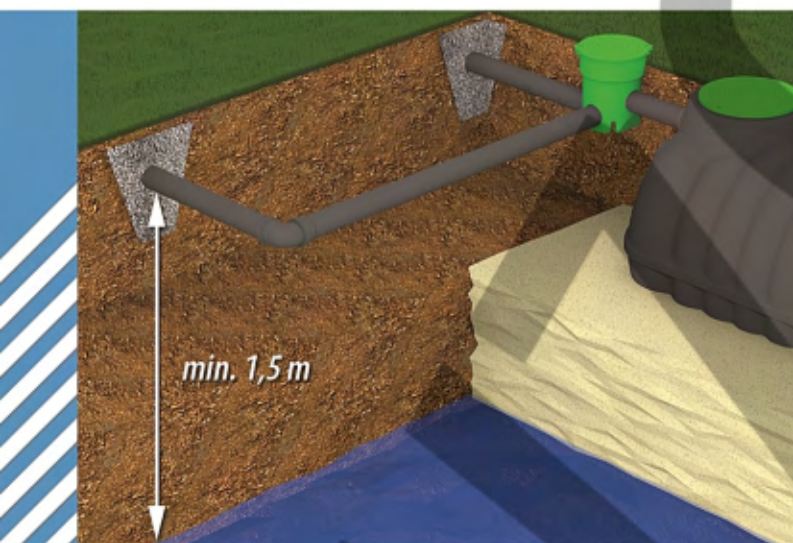
Rys. 6. Odległość ochronna / Drenaż rozsączający
