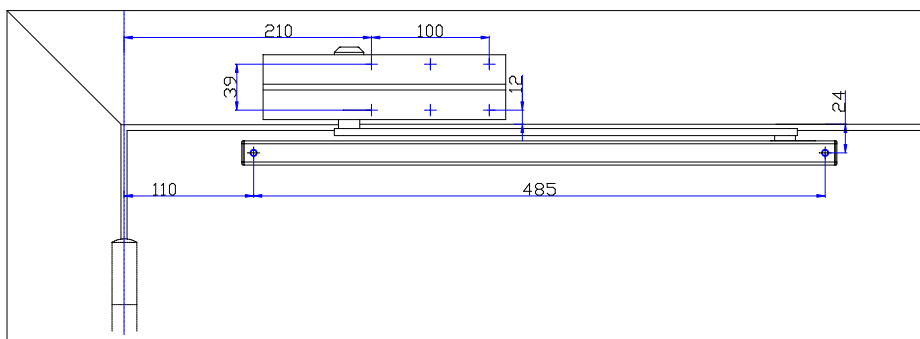
Montaż po stronie przeciwnej do zawiasów
