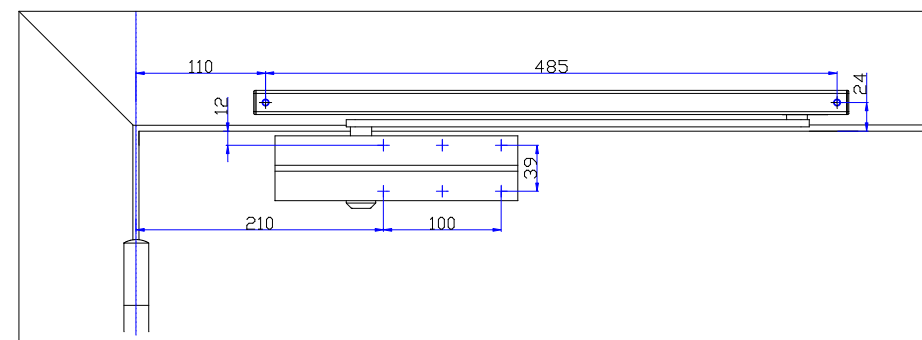
Montaż po stronie zawiasów
