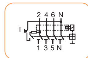
EFI-P4
