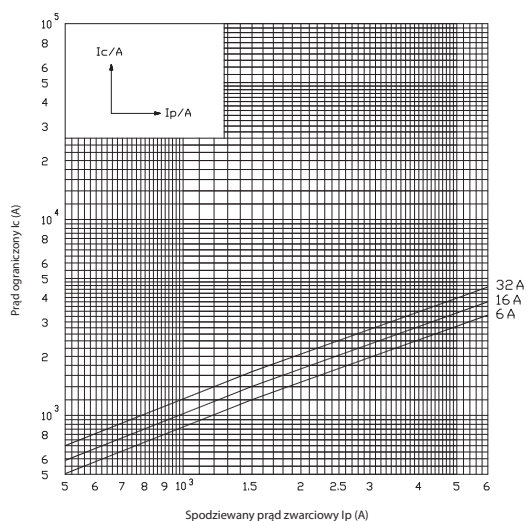
Charakterystyki prądów ograniczonych dla I_n = 6 A, 16 A, 32 A
