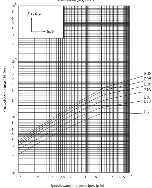
Charakterystyki I^2t
