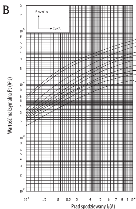
Charakterystyki całek wyłączenia I^2t wyłączników - charakterystyki B, C, D, K
