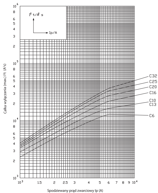
Charakterystyki prądów ograniczonych dla I_n = 6 A, 16 A, 32 A
