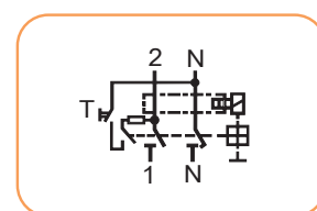
EFI-P2
