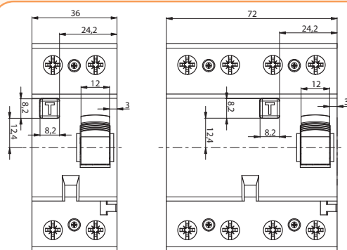
EFI-P2 16-80 A
