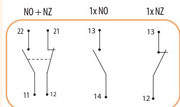
Układ styków
