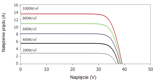
Wykres prądu w funkcji napięcia (54HL4R-B 445W)
