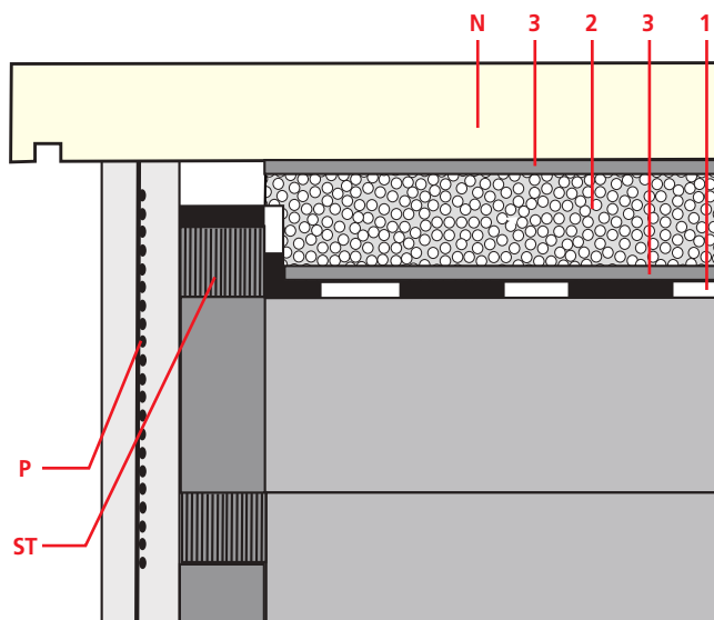
Przekrój warstw.
